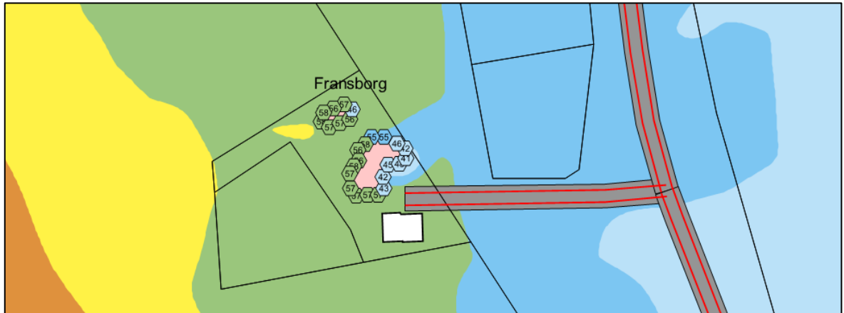
Figur 9. Urklipp från bilaga 5. Ekvivalent ljudnivå 2 m över mark samt vid fasad (högsta ljudnivån vid något våningsplan) från borring för sprängsalvor vid bostadsområde 3.
