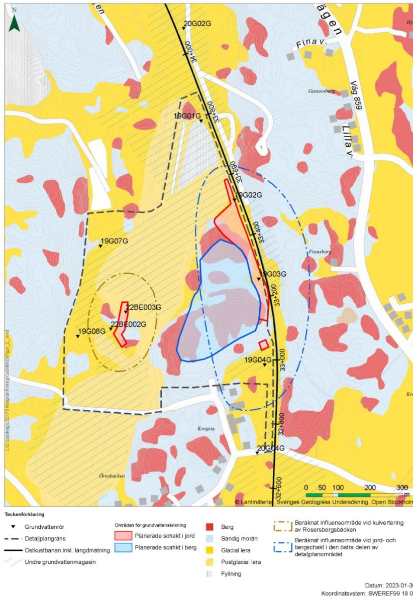
Figur 19 Bedömt influensområde för grundvatten till följd av planerad bergschakt (blått område) och schakt i jord (rött område).
