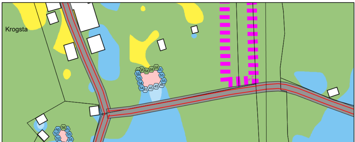
Figur 10. Urklipp från bilaga 5. Ekvivalent ljudnivå 2 m över mark samt vid fasad (högsta ljudnivån vid något våningsplan) från borring för sprängsalvor vid bostadsområde 5.
