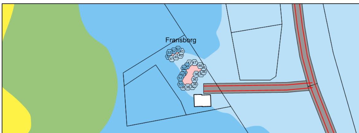
Figur 5. Urklipp från bilaga 2. Ekvivalent ljudnivå 2 m över mark samt vid fasad (högsta ljudnivån vid något våningsplan) från slagen spontning vid bostadsområde 3.
