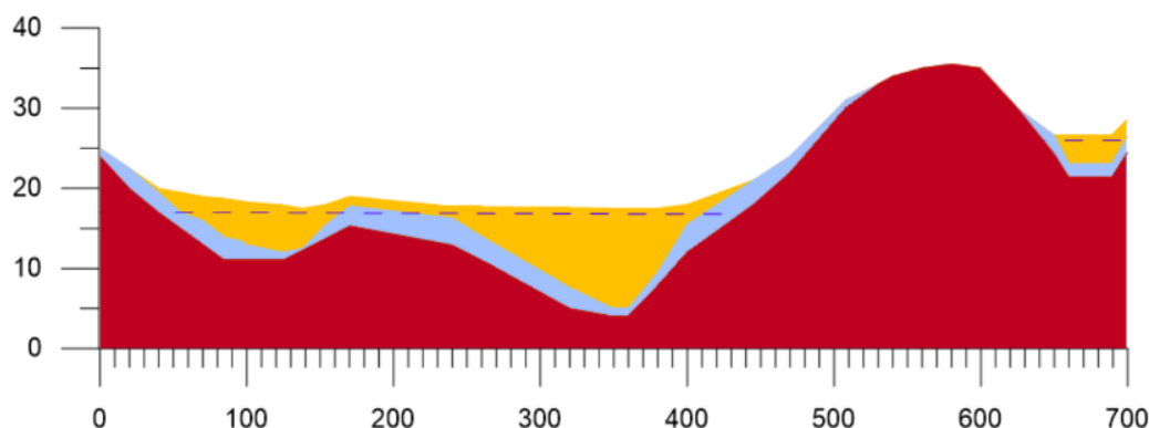
Figur 8 Tolkad jordlagerprofil från väster mot öster. Se blå markering i figur 6 för längdmätning. Bergab 2020-03-31.
