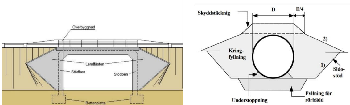
Figur 17 Till vänster exempel på plattramsbro. Till höger exempel på rörbro.
