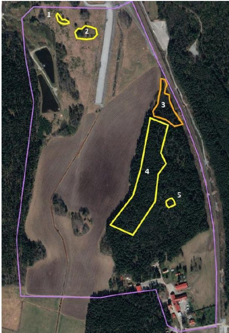
Figur 9 Identifierade naturvärden inom inventerat område (WSP 2018). Gul färg markerar områden med visst naturvärde och orange markerar område med påtagligt naturvärde. 1. Mindre åkerholme, 2. Större åkerholme, 3. F.d. sumpskog, 4. Barrskog, 5. Hällmarkstallskog.
