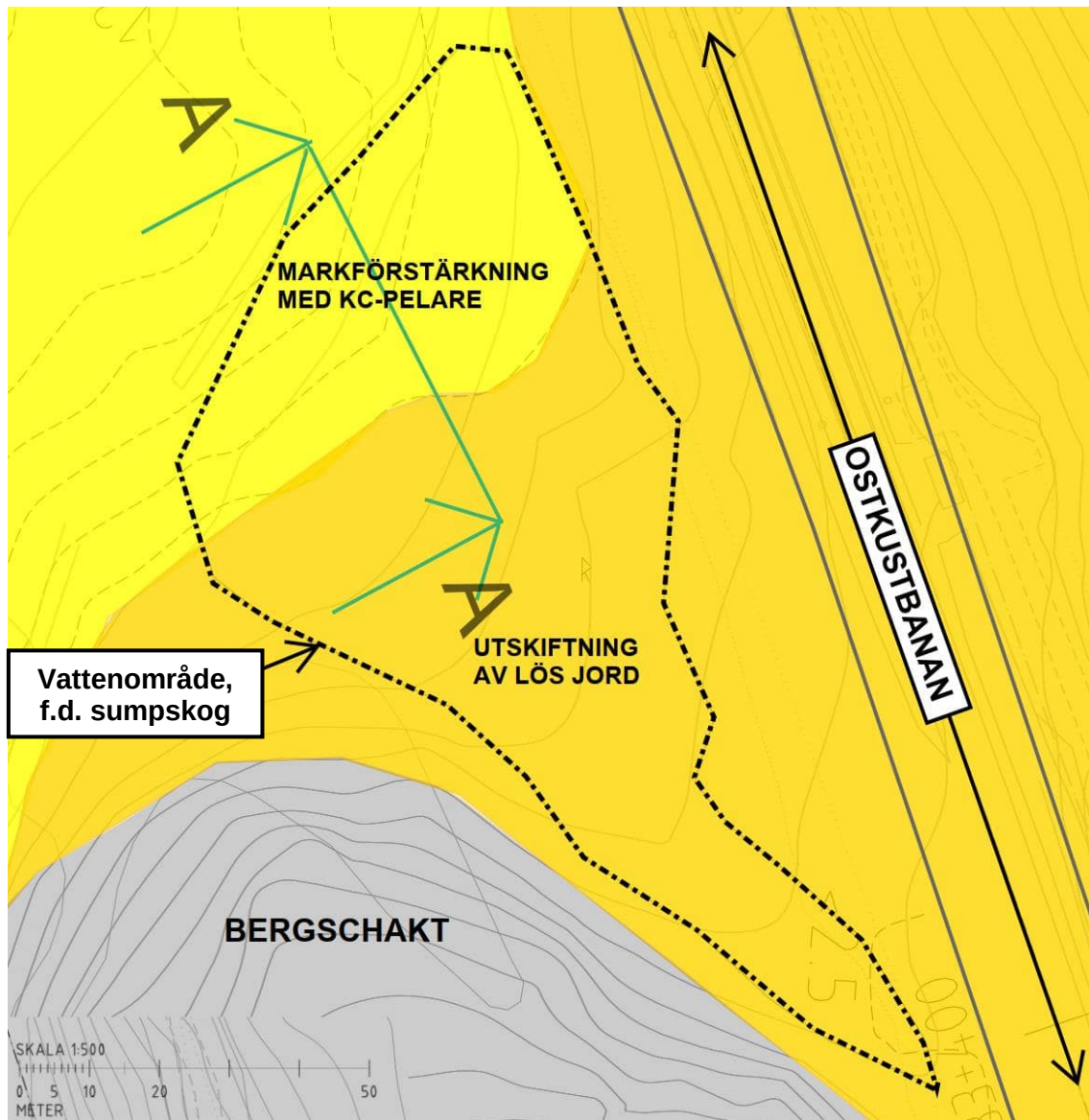
Figur 18 Planerade åtgärder inom befintligt vattenområde. I samband med utskiftning av lös jord kan även temporära grundvattensänkningar erfordras.
