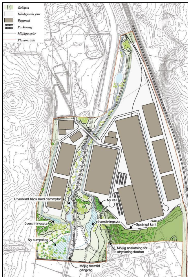
Figur 12 Illustrationsplan Brista verksamhetsområde (WSP 2019).
