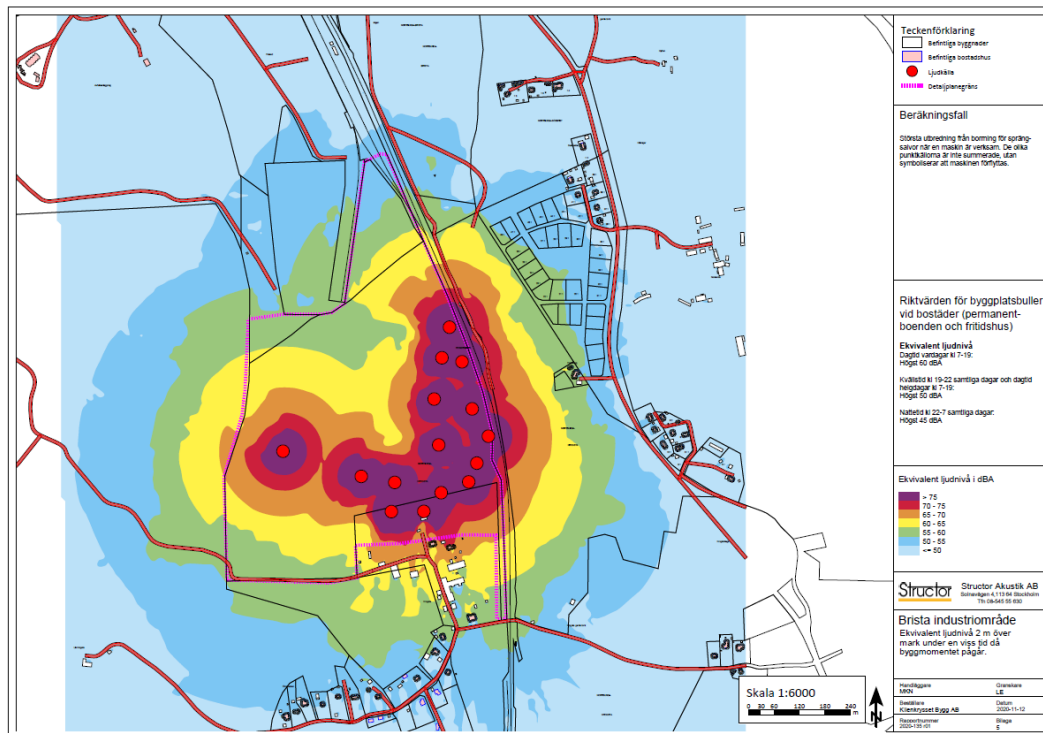
Figur 21. Beräknad utbredning av buller vid borring inför sprängning. Varje punkt representerar en plats där borring utförs.
