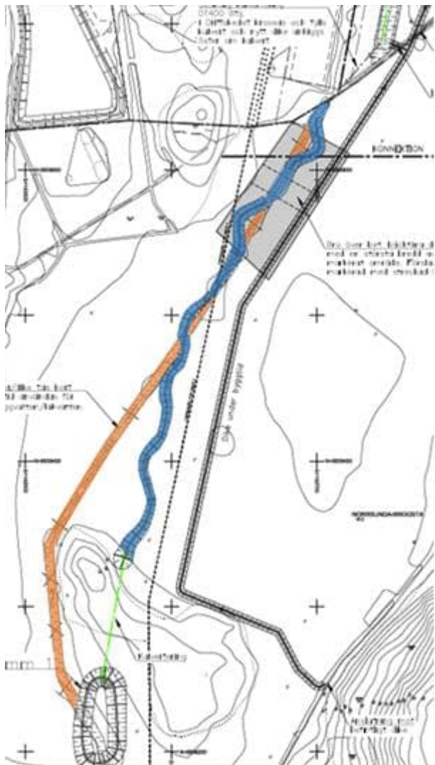
Figur 16 Ungefärlig utformning av planerad omläggning av Rosersbergbäcken. Inom blå ytor grävs ny bäckfåra. Orange ytor visar befintliga sträckor av bäcken som läggs igen efter att den nya bäckfåran gjorts klar.
