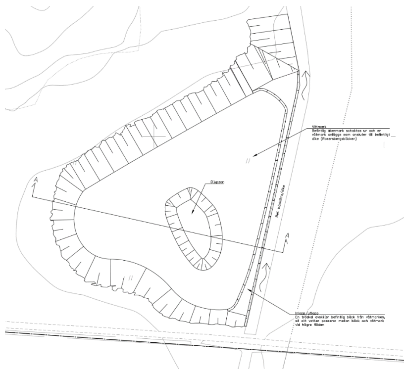
Figur 14 Tänkt våtmarksanläggning i anslutning till Rosersbergsbäcken.
