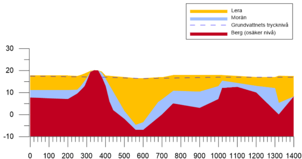
Figur 7 Tolkad jordlagerprofil från söder mot norr. Se röd markering i figur 6 för längdmätning. Bergab 2020-03-31.
