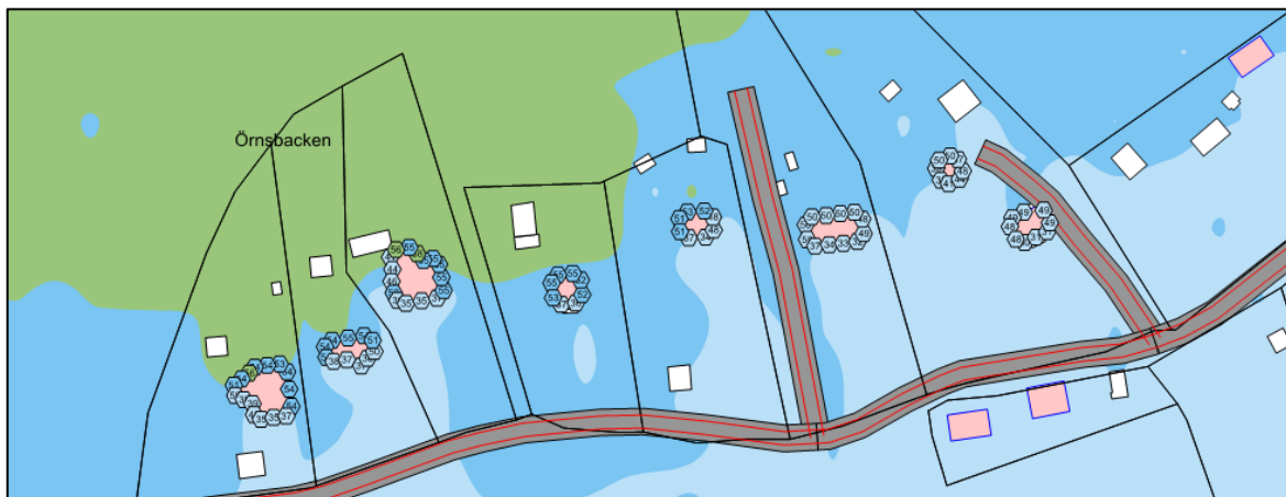
Figur 4. Urklipp från bilaga 1. Ekvivalent ljudnivå 2 m över mark samt vid fasad (högsta ljudnivån vid något våningsplan) från slagen pålning vid bostadsområde 6.
