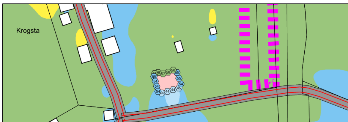
Figur 7. Urklipp från bilaga 3. Ekvivalent ljudnivå 2 m över mark samt vid fasad (högsta ljudnivån vid något våningsplan) från bergschakt vid bostadsområde 5.
