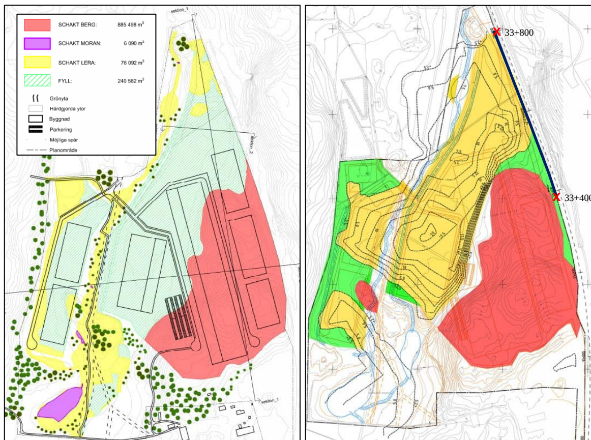
Figur 3. T.V. Mängdning färgkarta (WSP, 2019-09-16). T.H. Detaljplaneområde med tolkade lerdjupskurvor med översiktligt bedömt förstärkningsbehov med avseende på grundläggning. Röda områden: byggnader grundläggs med plattor på berg. Gröna områden: byggnader grundläggs med pålar alternativt med plattor på packad fyllning efter utgrävning av lös jord. Gula områden: byggnader grundläggs med pålar. Spontning planeras ungefär utmed blå linje . Ritningen är hämtad från "PM Geoteknik, Brista, dat. 2019-10-01".
