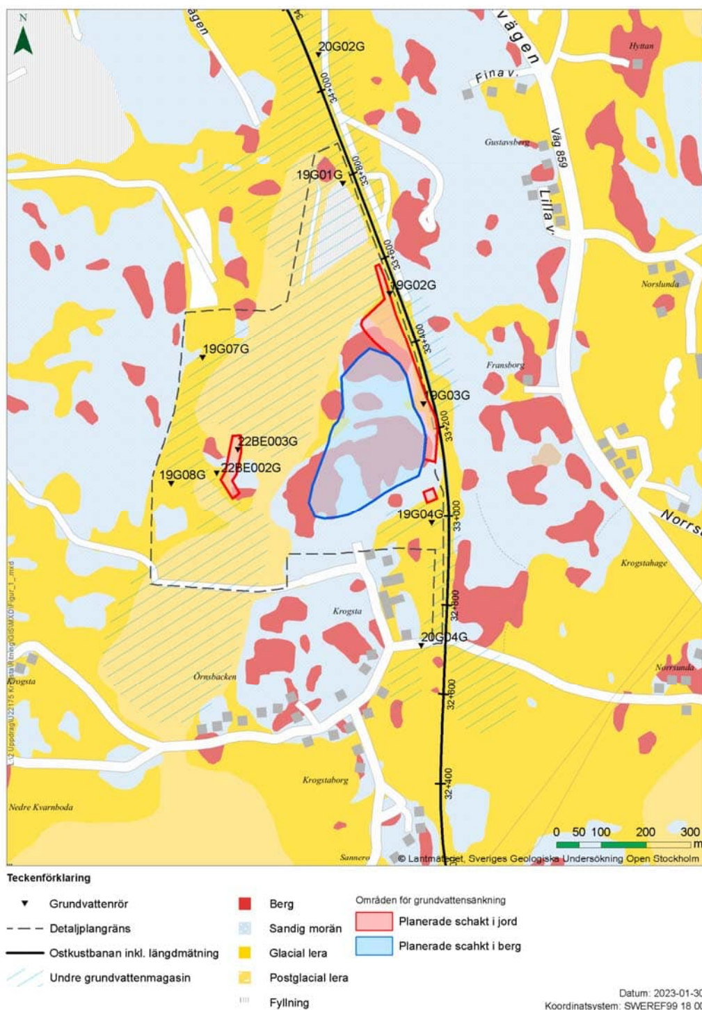
Figur 1. Planerade schakt inom planområdet som kan medföra tillfällig grundvattenbortledning (enligt Teknisk beskrivning 2022-03-16 figur 31 och dess Bilaga 1).
