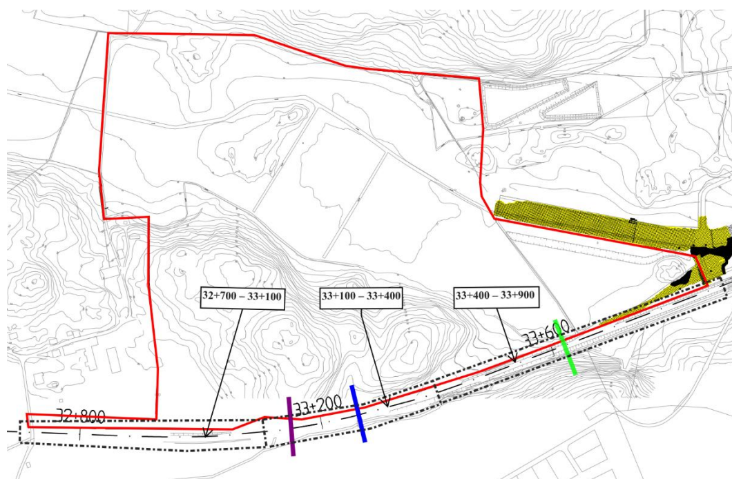
Figur 10. Översikt med Ostkustbanans längdmätning i vy mot väster (norr till höger i bilden). Gulrastrerade områden illustrerar befintliga markförstärkningsåtgärder.
