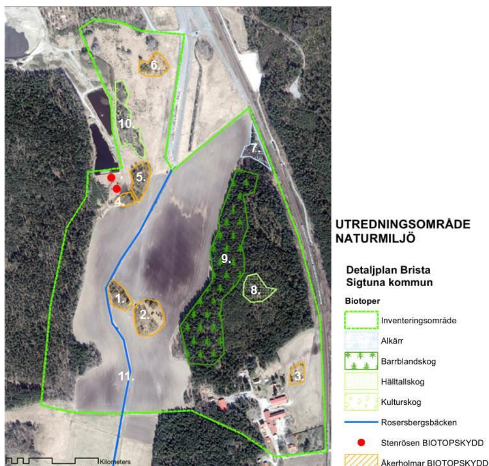
Figur 10. Översikt av de biotoper som bedömts ha naturvärden. Se även Bilaga 1.
